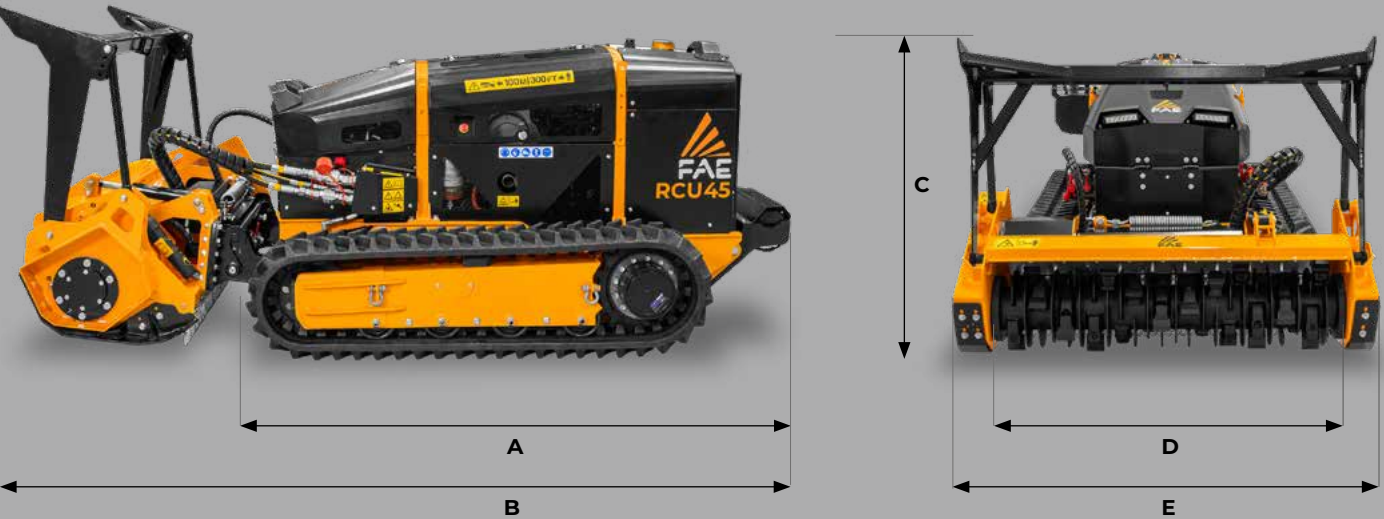
A Lunghezza totale senza attrezzatura 1970 mm B Lunghezza di trasporto con testata BLO/RCU a terra 3090 mm C Altezza massima 1120 mm D Largh. esterna cingoli 1300 mm E Vedi tabella testate
