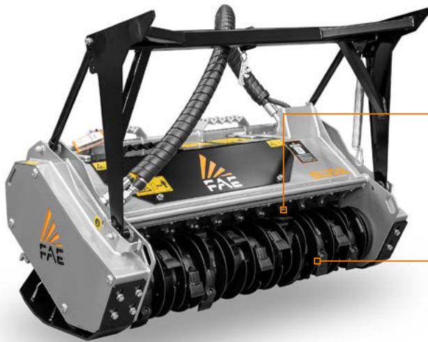
Rotore con tecnologia Bite Limiter massima produttività e minima richiesta di potenza grazie agli speciali inserti in acciaio altamente resistente e alle lame di tipo BL/MINI
