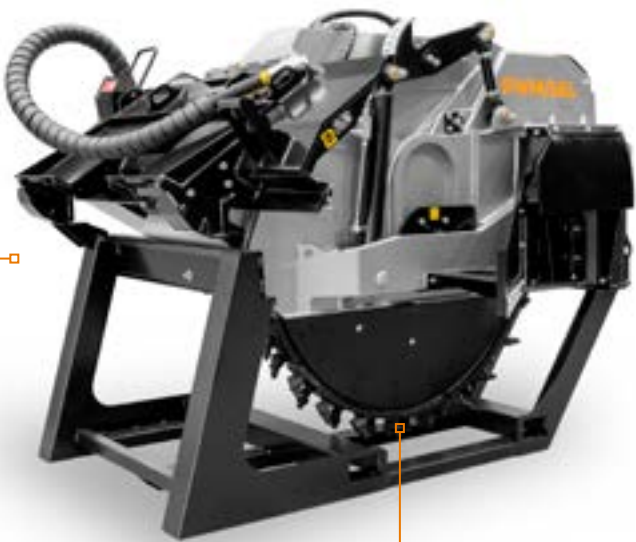
Slitte autolivellanti con controllo idraulico della profondità
