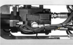
Motore idraulico ad ingranaggi da 16 cc con valvola anticavzionale integrata - (35 - 40 L/min)
