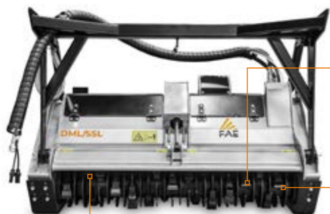
Rotor avec technologie Bite Limiter productivité maximale et demande de puissance minimale grâce aux inserts spéciaux en acier haute résistance et aux lames de type BL/MINI (DML/SSL/BL et DML/SSL/BL/SONIC)
