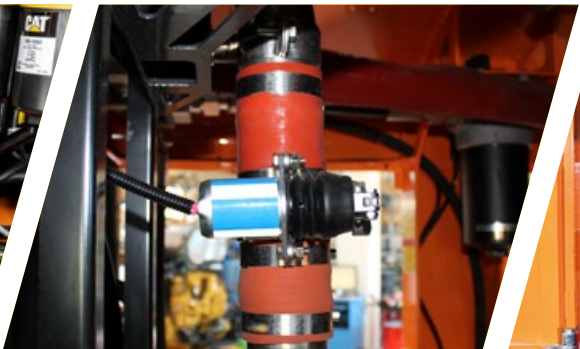
Sistema air shut-off
