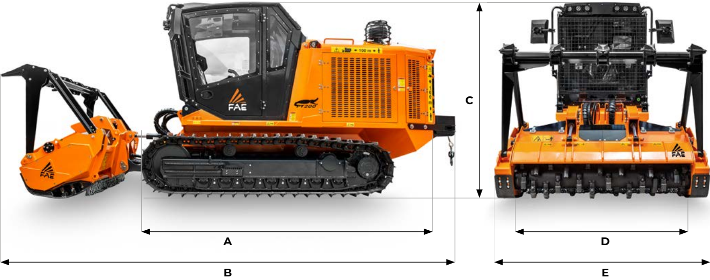
A Gesamtlänge ohne Anbaugerät B Transportlänge mit Seilwinde und 140/U/PT Anbaugerät am Boden 4518 mm 6422 mm C Max. Höhe D Spur Gesamtbreite E Siehe Anbaugeräte-Tabelle 2654 mm 2050 mm (mit 500 mm Stegplatten)
