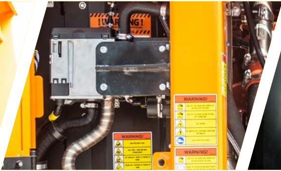
System zum Vorwärmen von Motor und Hydrauliköl
