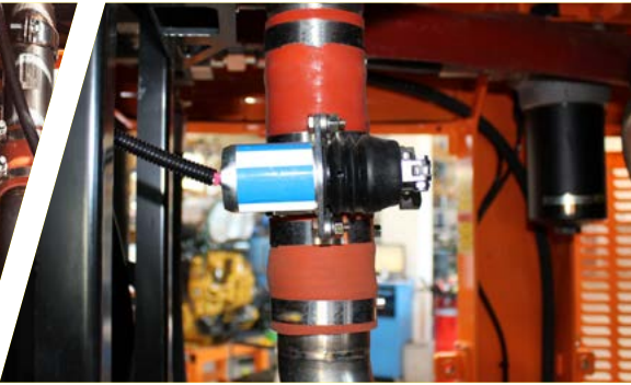
Air Shut-Off Sicherheitsventil
