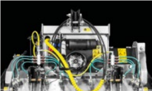
Das Water Spray System dient sowohl zum Kühlen als auch zum Mischen
